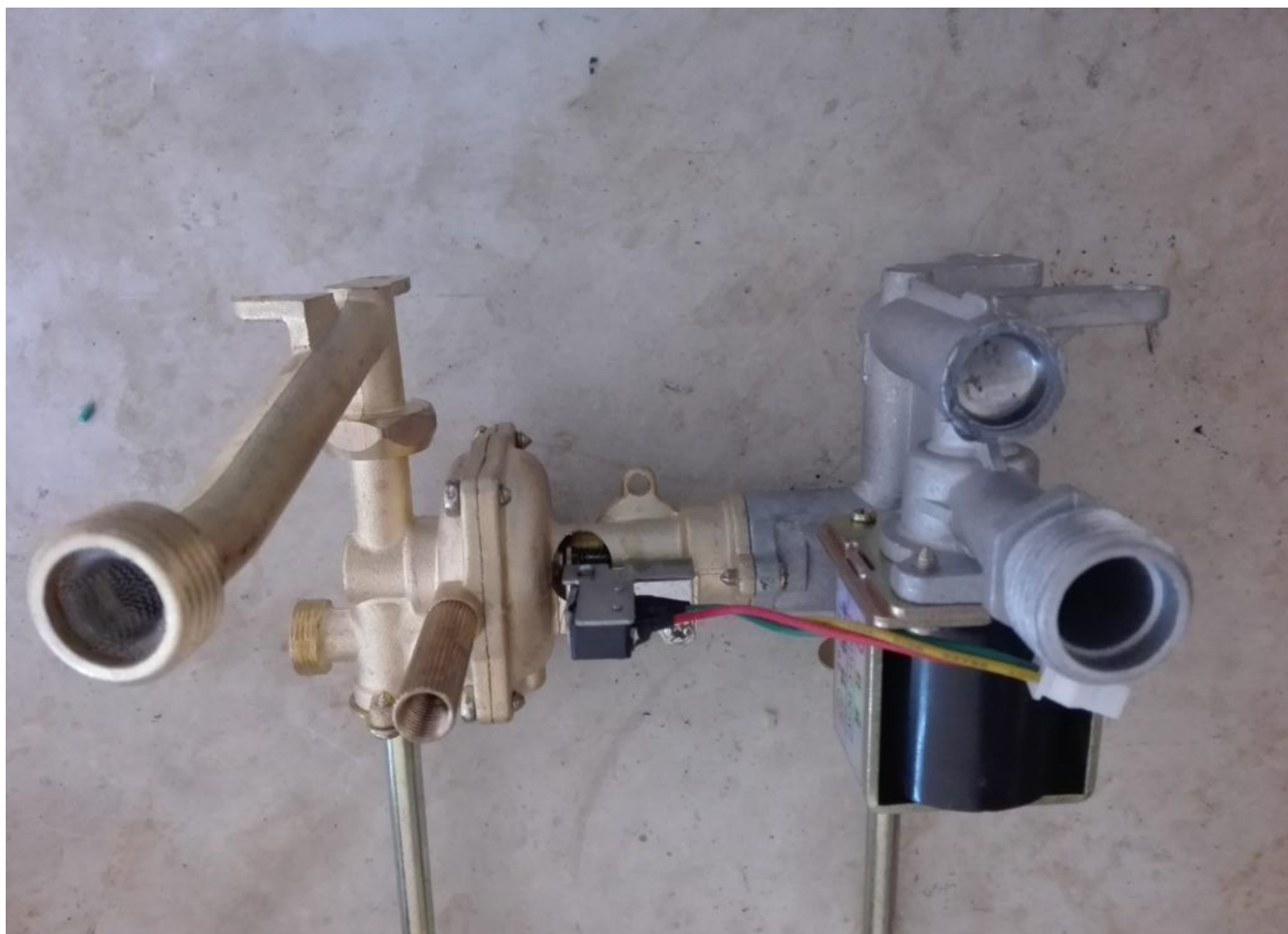
Core Mécanique du chauffe-eau Electronique 10 litre
