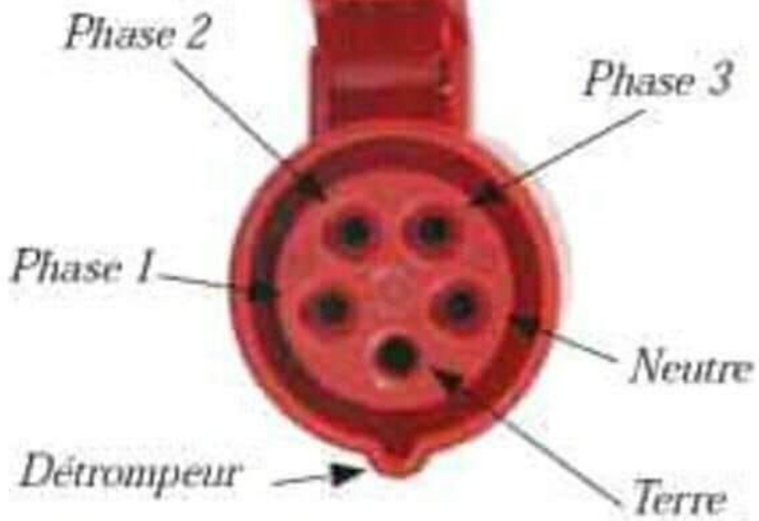
Prise femelle triphasée vue extérieure.
